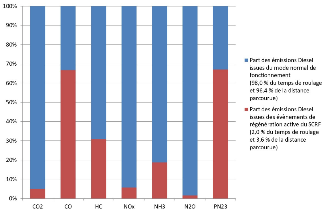
Emissions du véhicule diesel : contribution (en rouge) des régénérations actives du filtre à particules à la totalité des émissions
