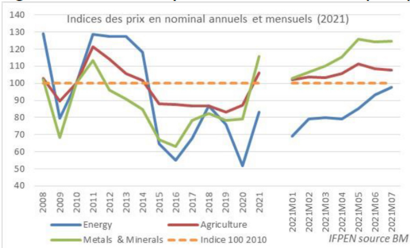
Figure 12 : Indices des prix annuels et mensuels (2021)
