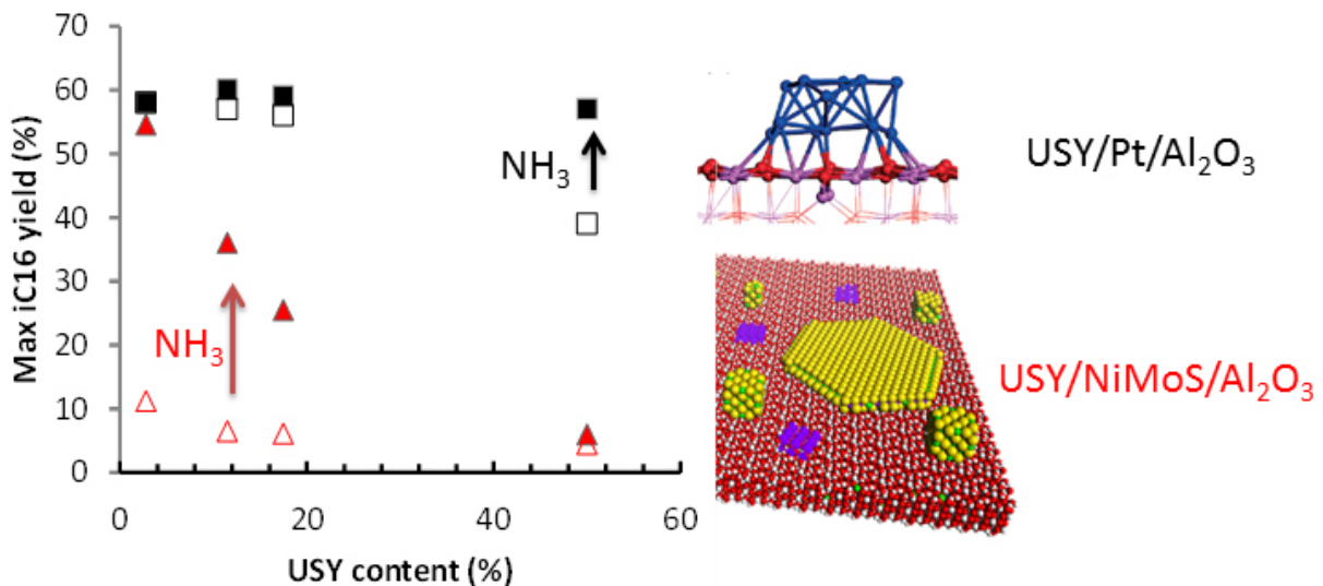
Figure 2 : Comparaison des catalyseurs bifonctionnels au Pt (noir) ou Ni/MoS2 (rouge). La concentration des sites acides a été modifiée en faisant varier la teneur en zéolithe USY dans l'extrudé. La figure montre le rendement maximal en iC16, en présence (symboles pleins) ou absence (symboles vides) d'ammoniaque comme inhibiteur.
