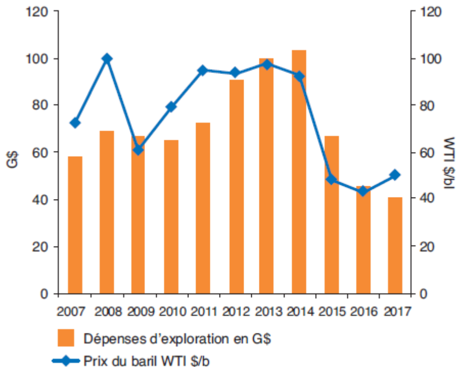
Fig. 1 – Évolution des dépenses d’exploration et du prix du baril WTI entre 2007 et 2017
